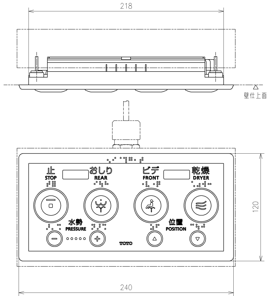
リモコン詳細図
